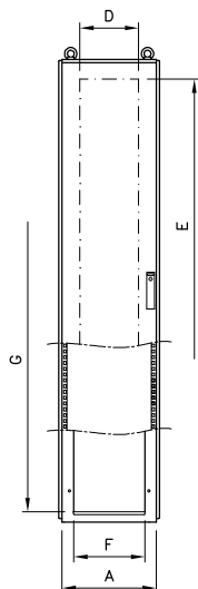
"RXP" Porta anteriore
