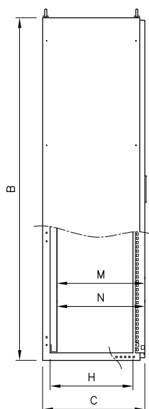
Module with double blind door
