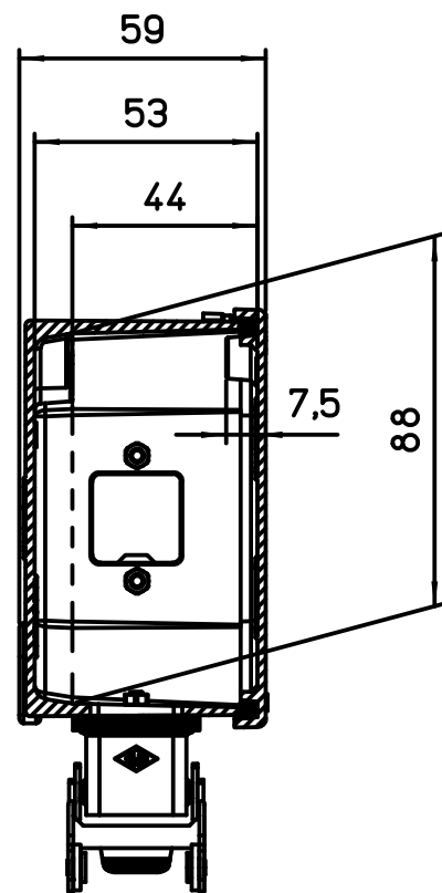
Sez. A-A
