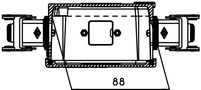
Sez. B-B
